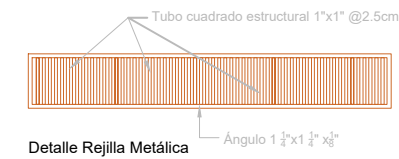
Detalle Rejilla Metálica
