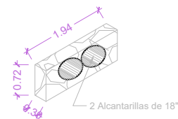
Detalle cabezal Mampostería
