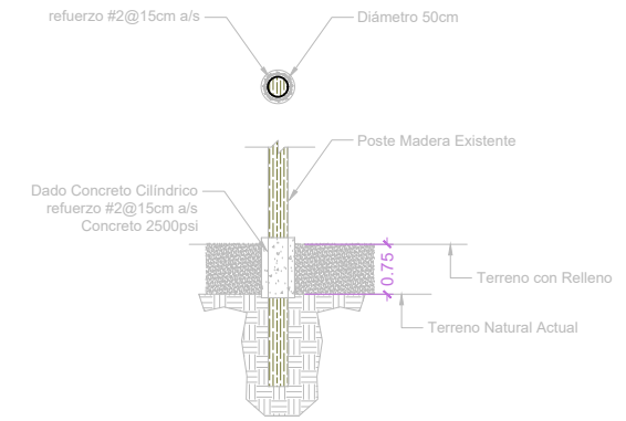
Detalle dado de Concreto Cilíndrico
