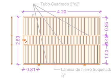
Detalle portón vehicular
