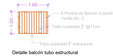
Detalle balcón tubo estructural
